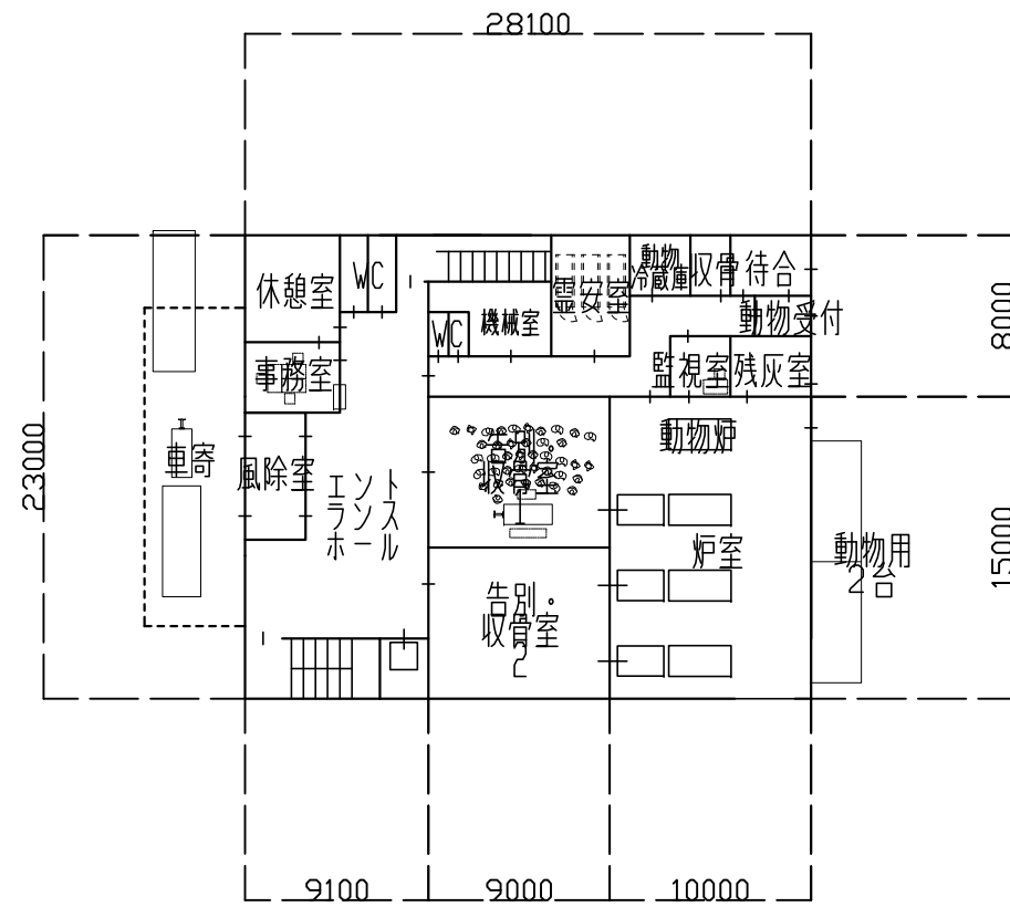
1階平面図
