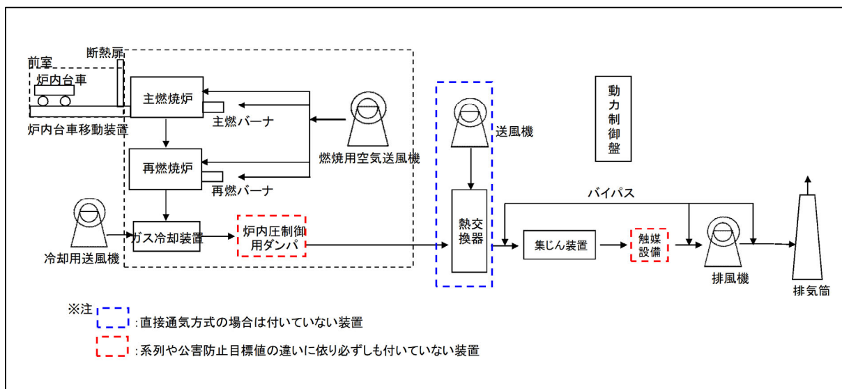
図7-1 火葬炉設備の構成フロー
