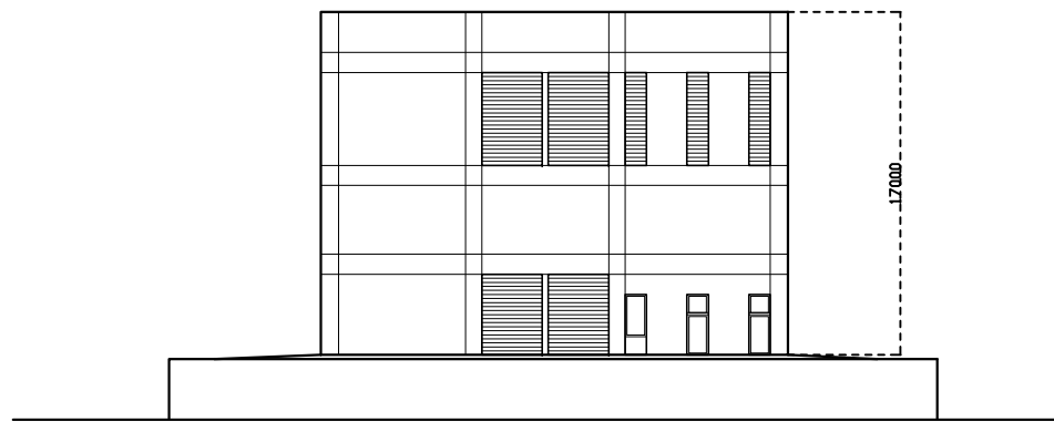
北立面图
