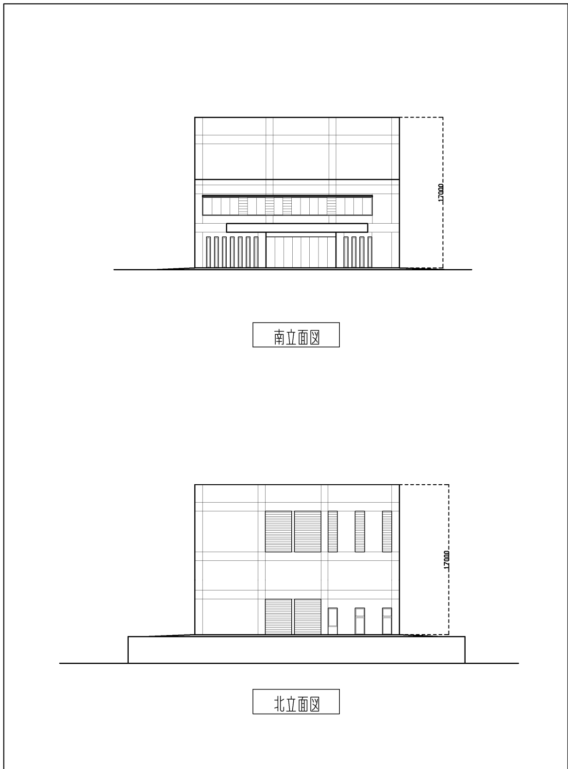
図6-7 立面計画案（南、北）
