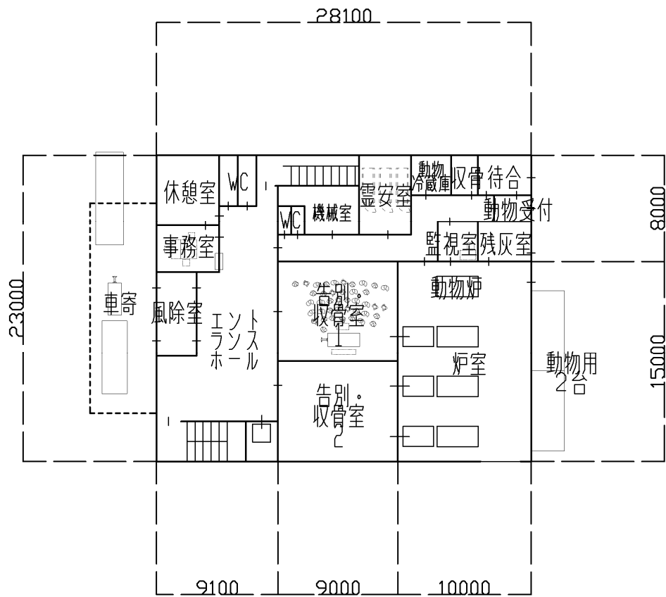
1階平面図
