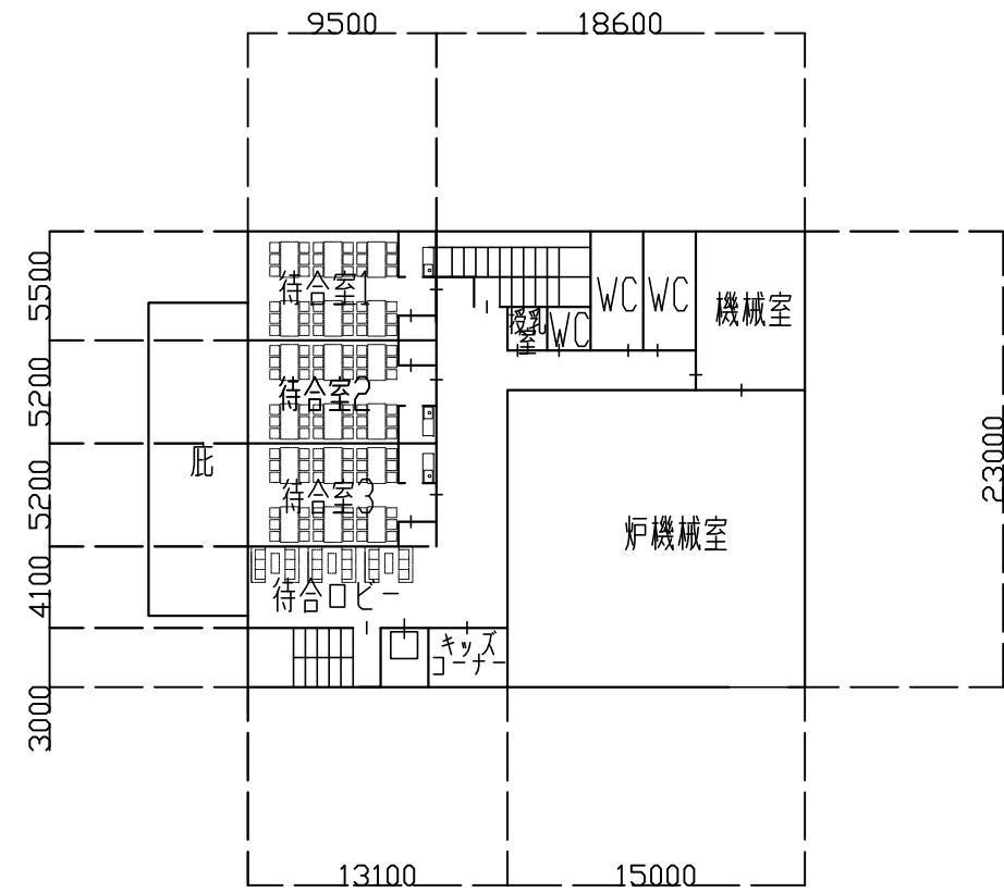
2階平面図
