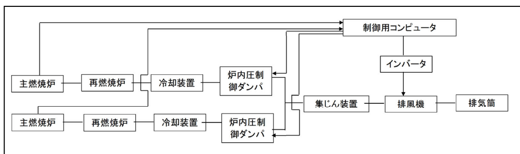
図 7-4 炉内圧力制御システムの概要
