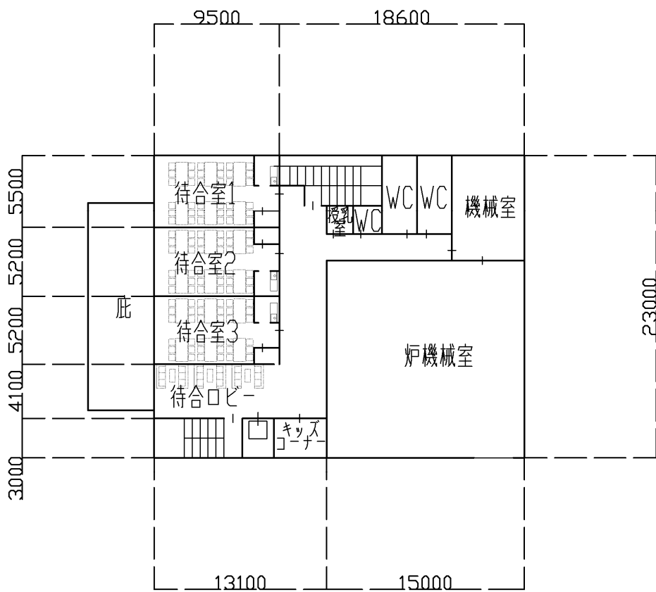
2階平面図
