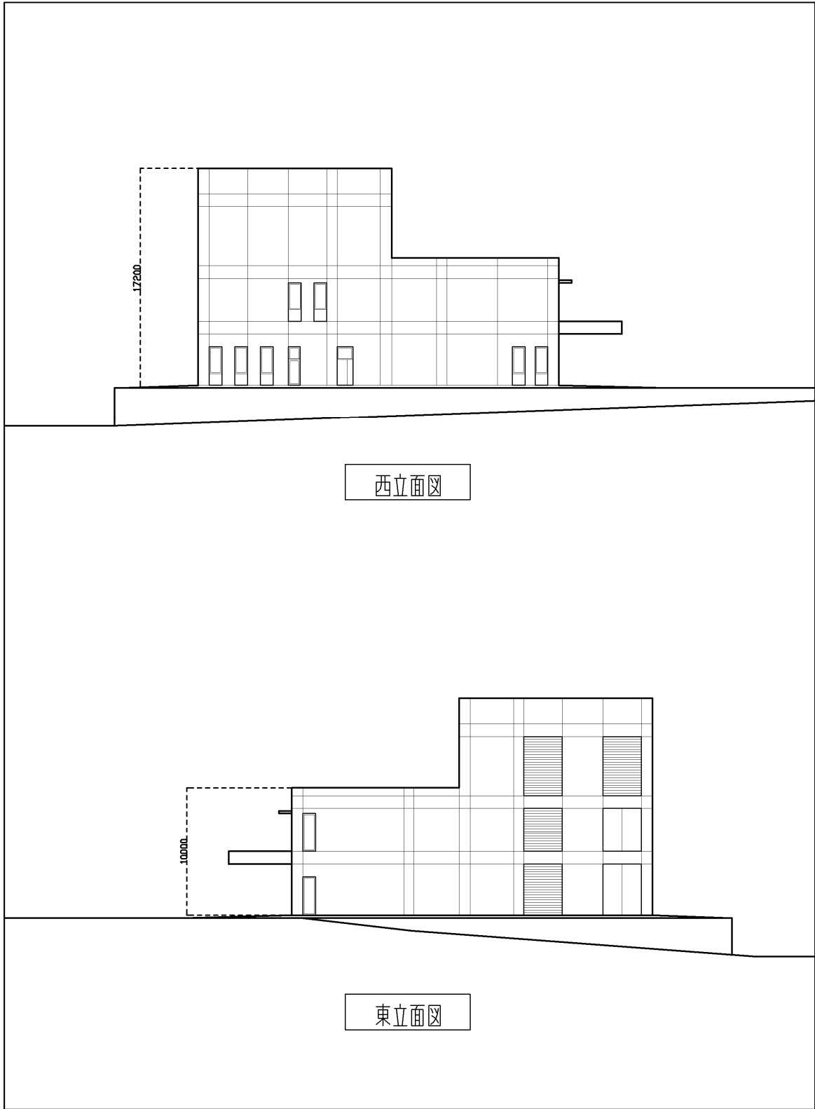
图 6-8 立面計畫案 (西、東)
