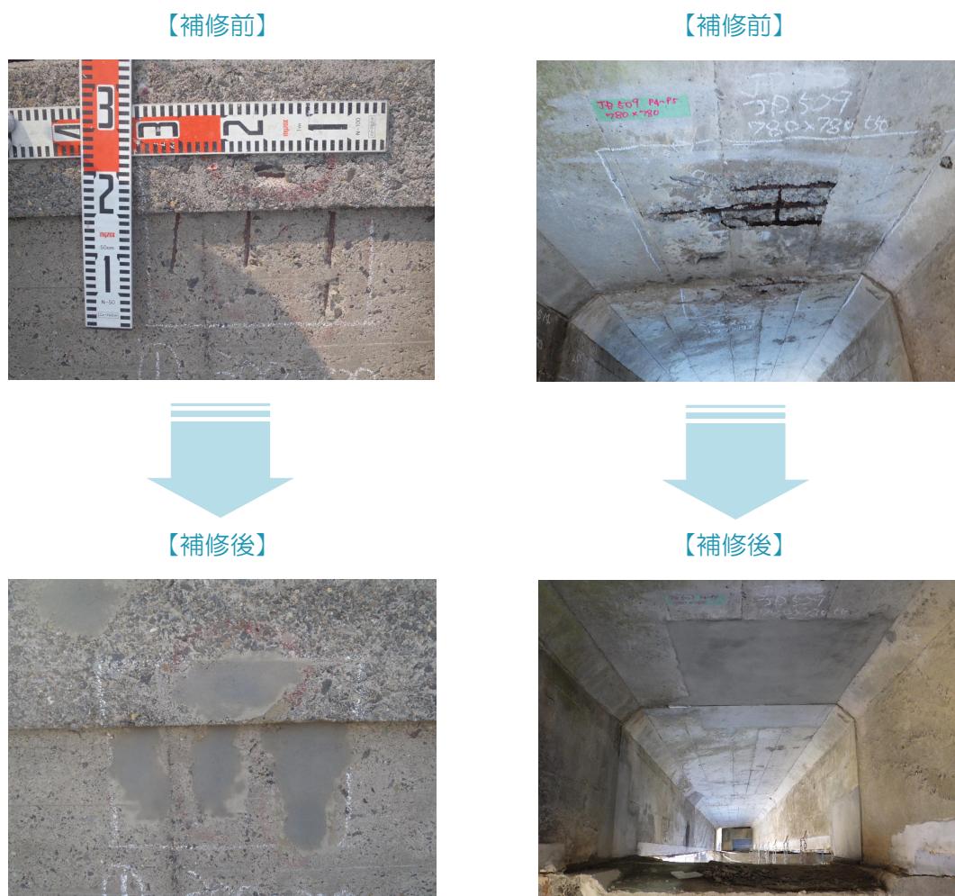
図 3 橋梁補修例
